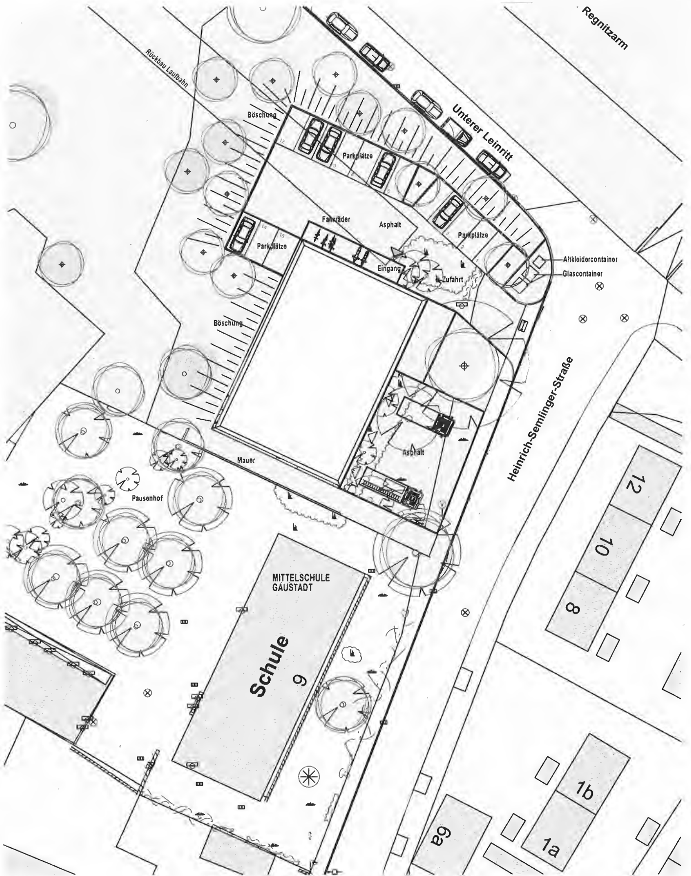
Neubau eines Feuerwehrgerätehauses für die Löschgruppe 5 - Lageplan
